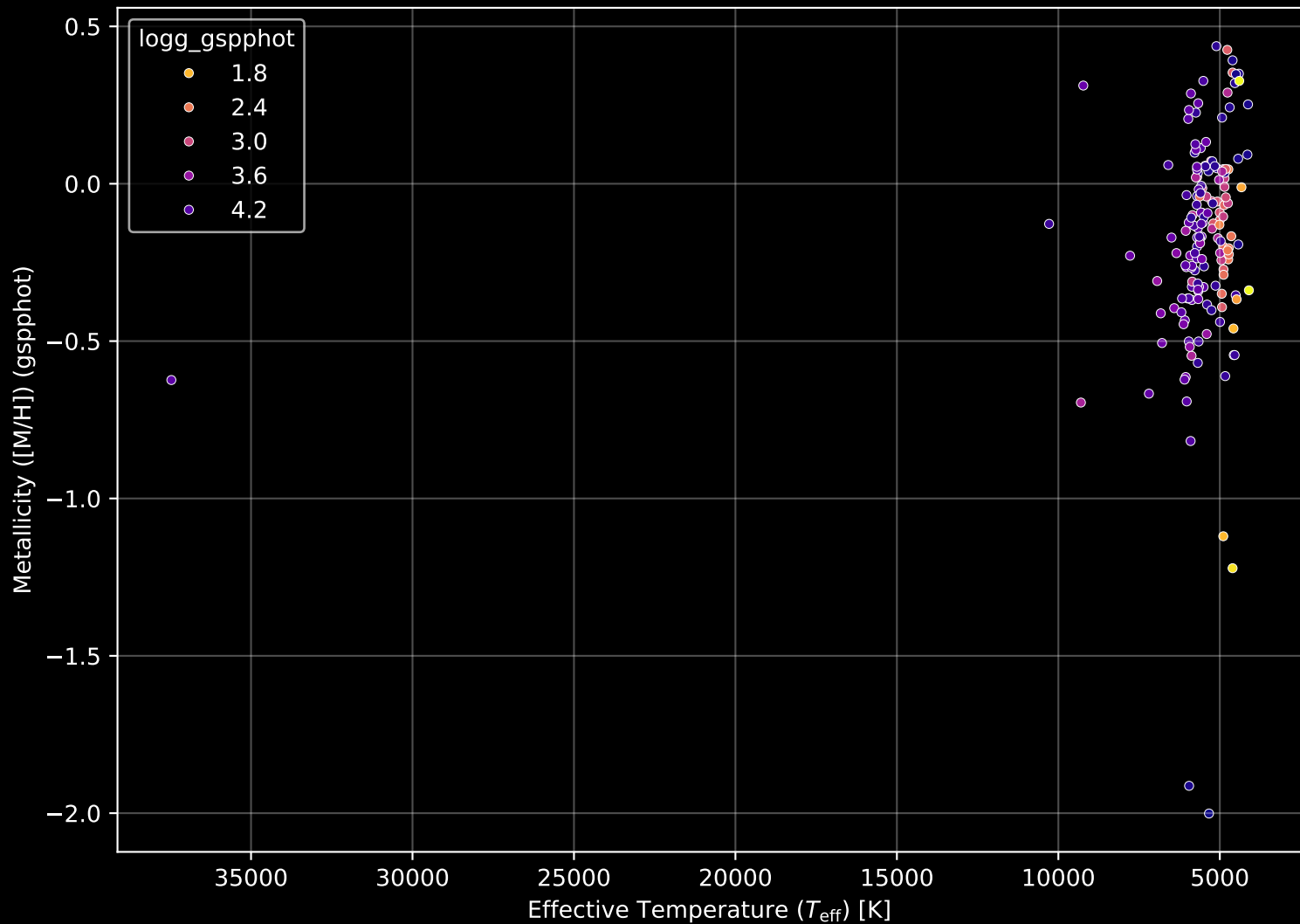
APOGEE DR17 Field: [273-30-O_TESS] Stellar Population Parameters (n= 165)
